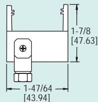
Switch Module
